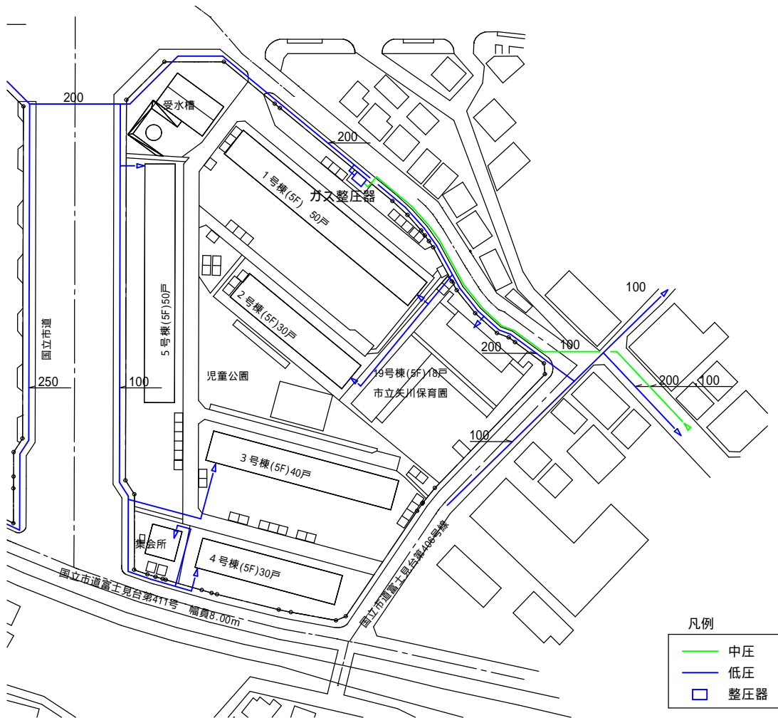
矢川公共用地のガス設備参考図
