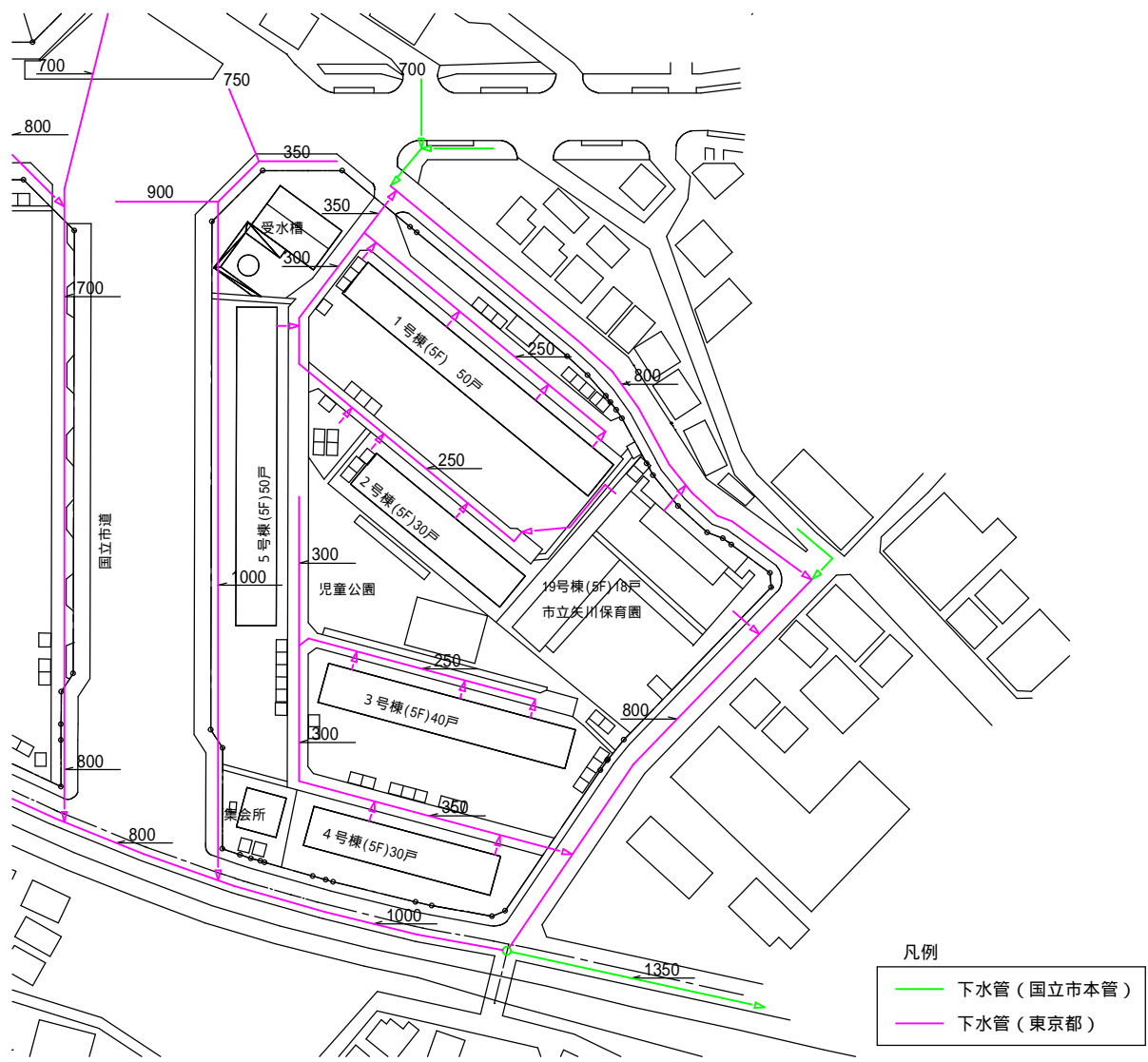
矢川公共用地の排水設備参考図
