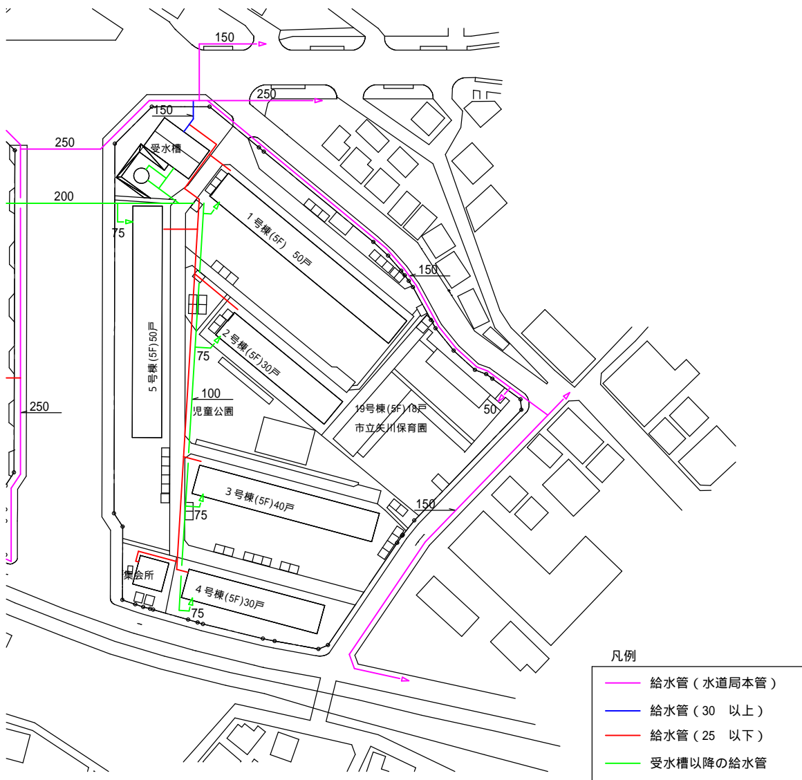
矢川公共用地の給水設備参考図
