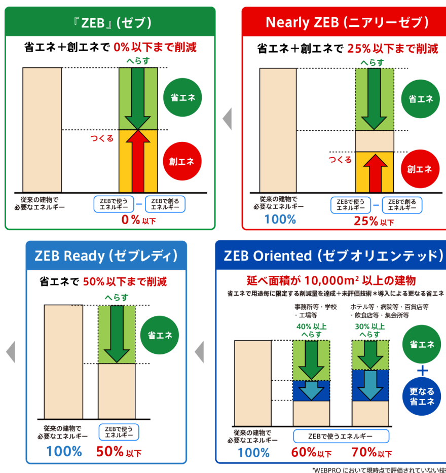
図表 50 ZEBの種類と定義
