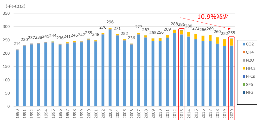
図表 23 国立市の温室効果ガス排出量の推移
