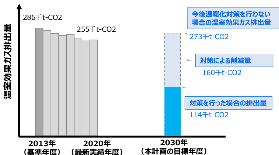
図表 40 2030 年度の温室効果ガス排出量
