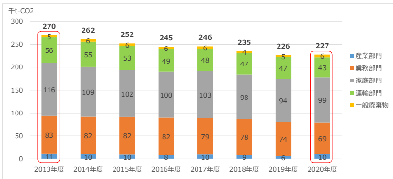
図表 26 国立市の部門別 CO2 排出量の推移
