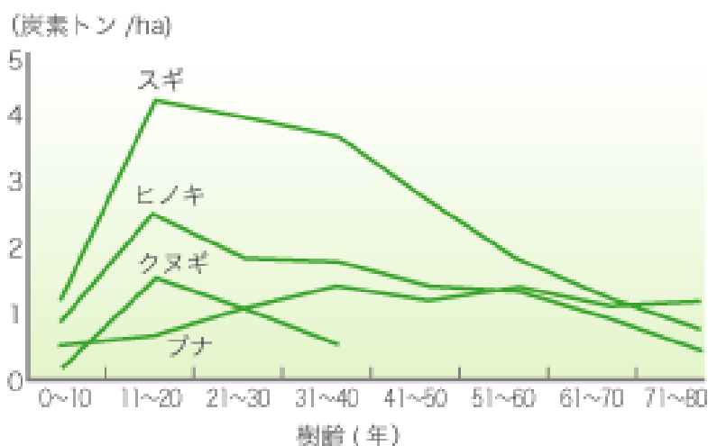
図表 35 樹種・林齢別炭素吸収量
