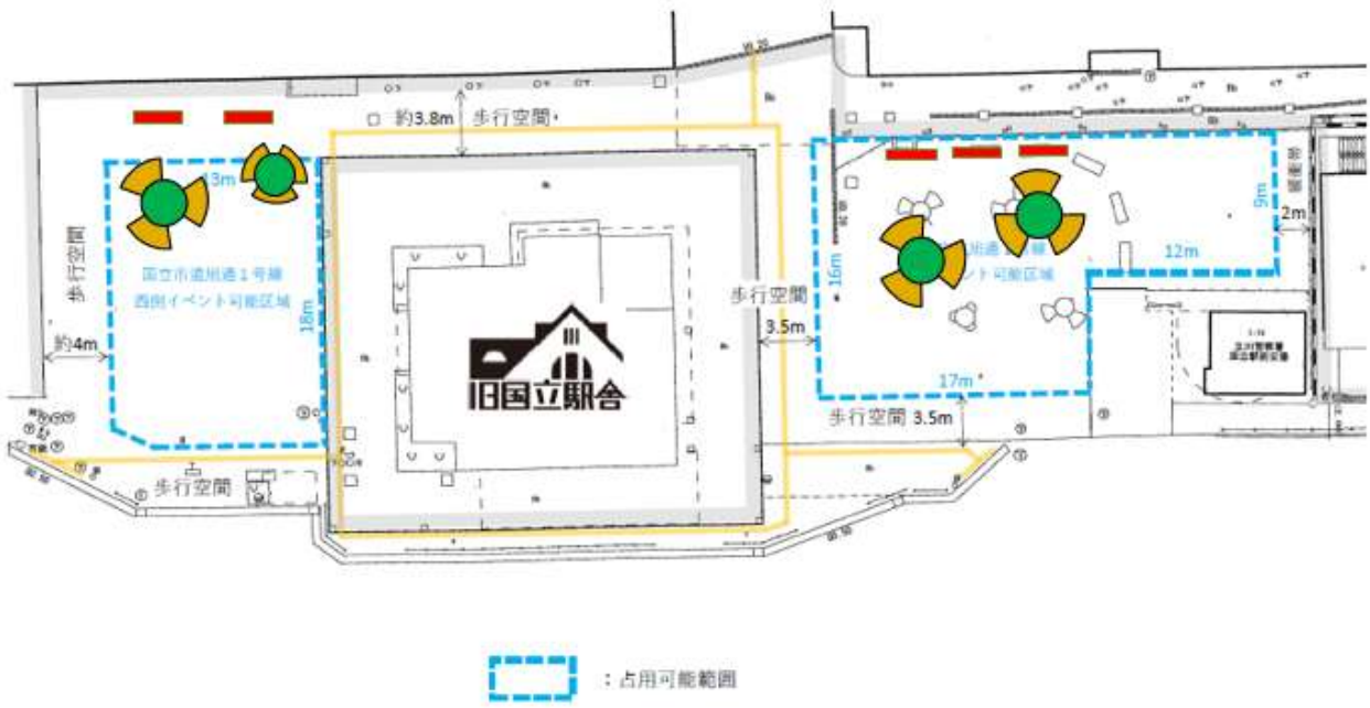
国立駅南口駅前広場 概略平面図 縮尺1/300 (A4判)
