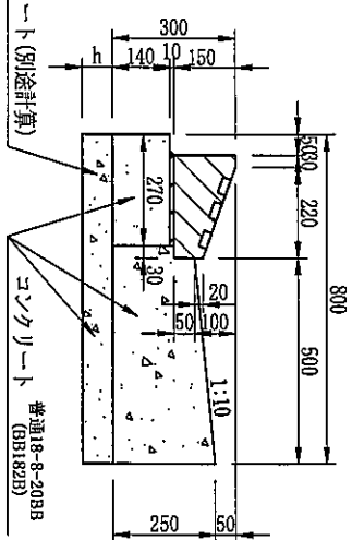
B-B 断面図
