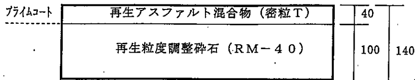
歩道アスファルト舗装（14型）（単位mm）
