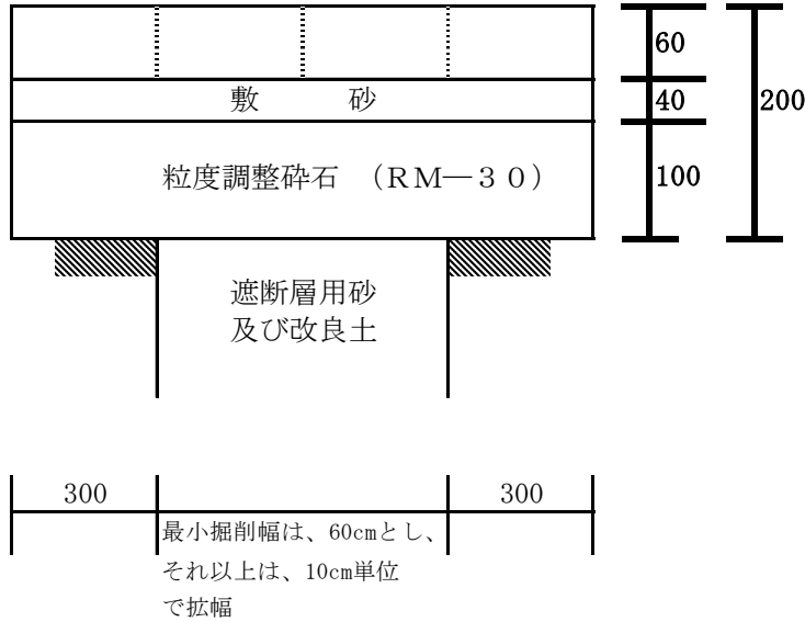
歩道平板舗装 (20型) (単位mm)
