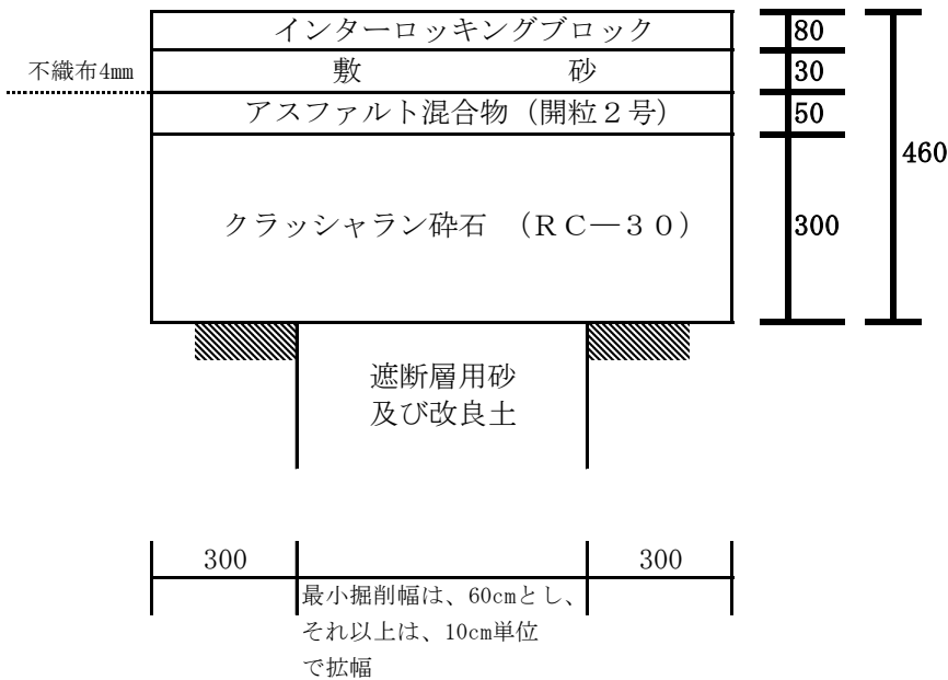
インターロッキング ブロック舗装 (46型) (単位mm)
