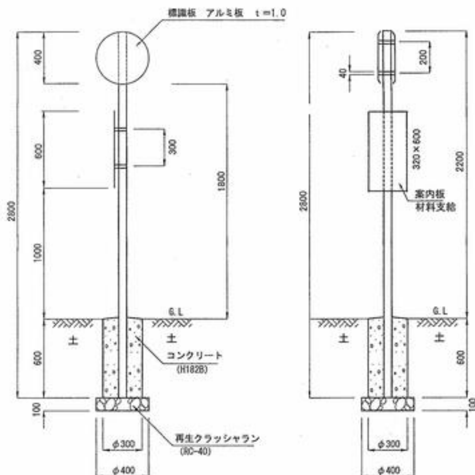
材 料 表 (停留所標識)
