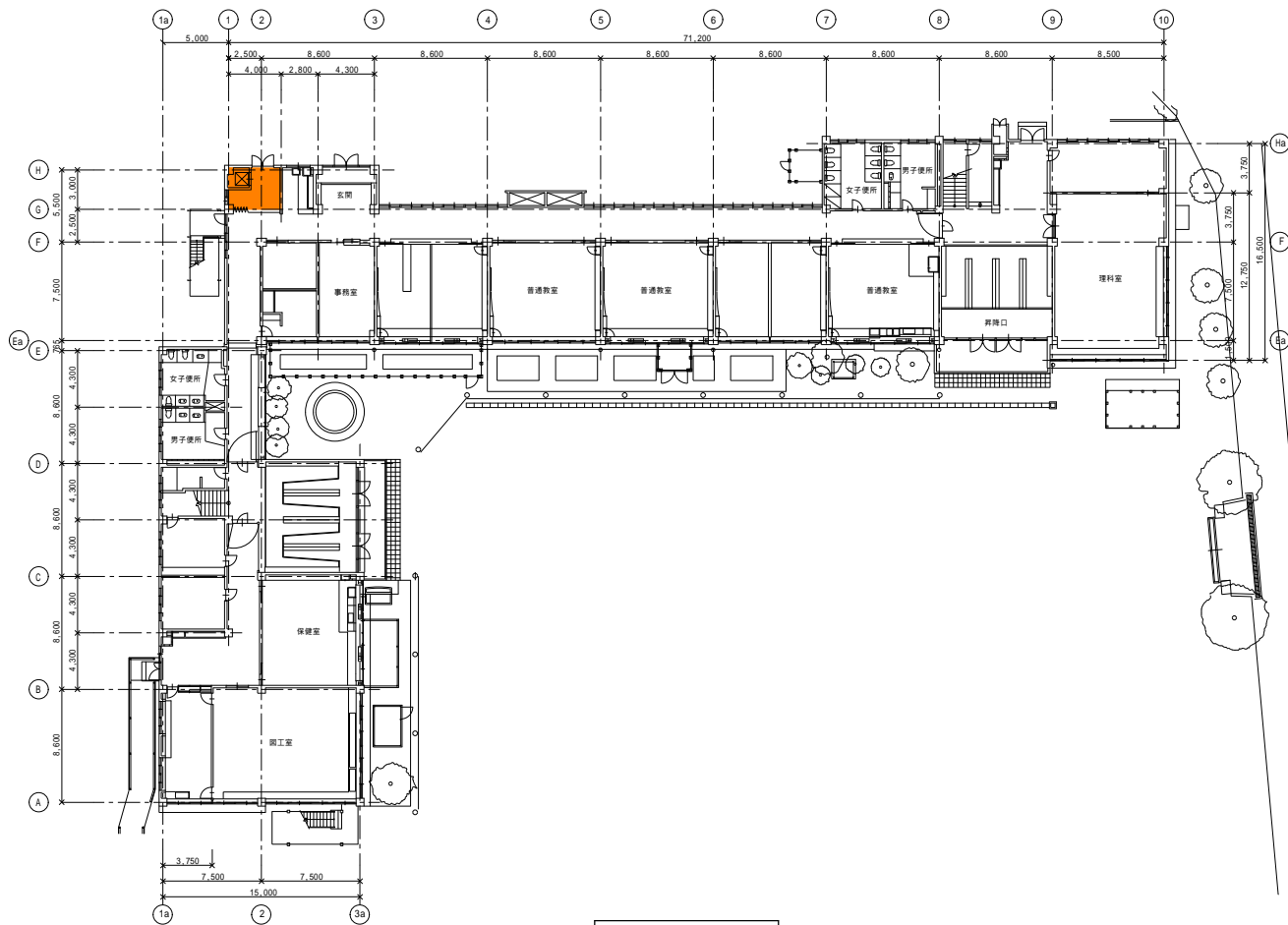
1 階 平 面 图
