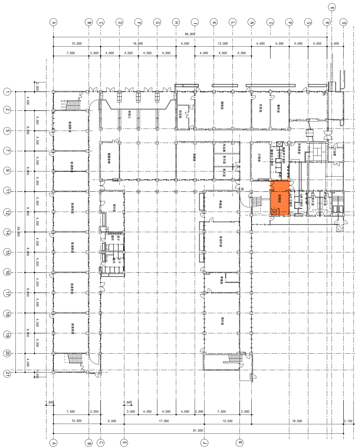
1 階平面図
