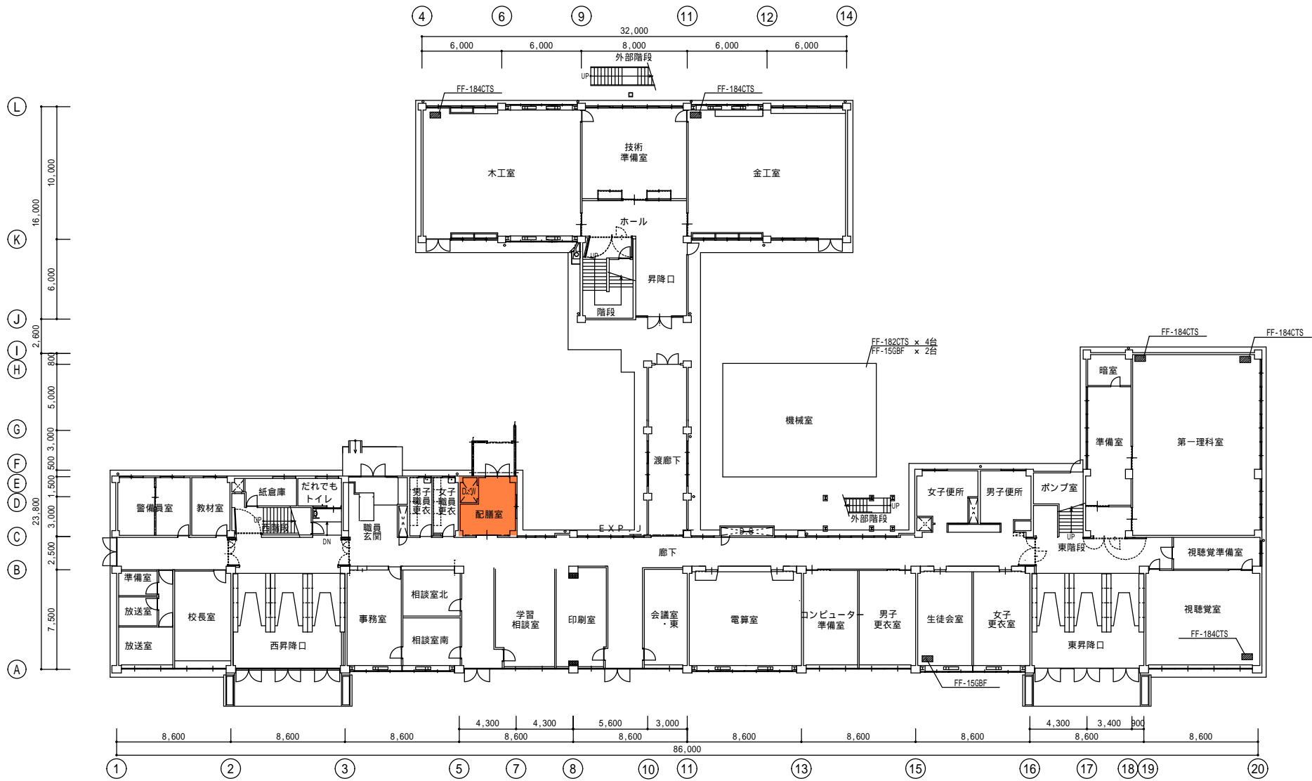
1階平面図1:200
